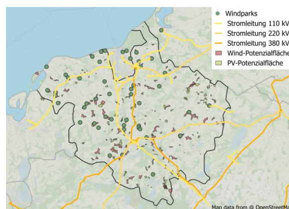
Abbildung 8: Strominfrastruktur (HS, HHS); EE-Potenzialflächen und Bestand Windkraftanlagen
