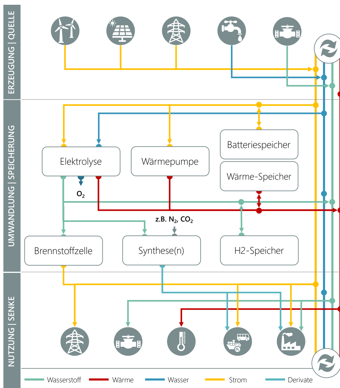
Abbildung 5: Ganzheitliche Betrachtung der Stoffströme von Erzeugung, über Umwandlung bis zur Nutzung
